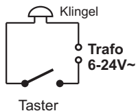
b) Installationsschema - Inbetriebnahme durch Spannungsaufgabe 6-24V~
